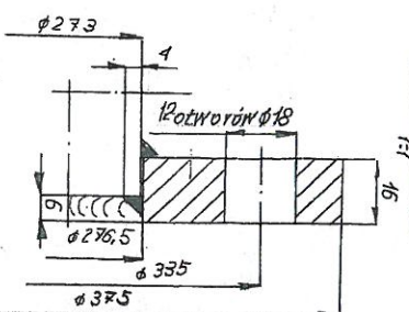
Szczegół. E'
